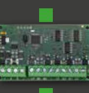
AUXI-A 10020069 5 zone/uitgangen of 4 spanningsgestuurde in/uitgangen (programmeerbaar) module
